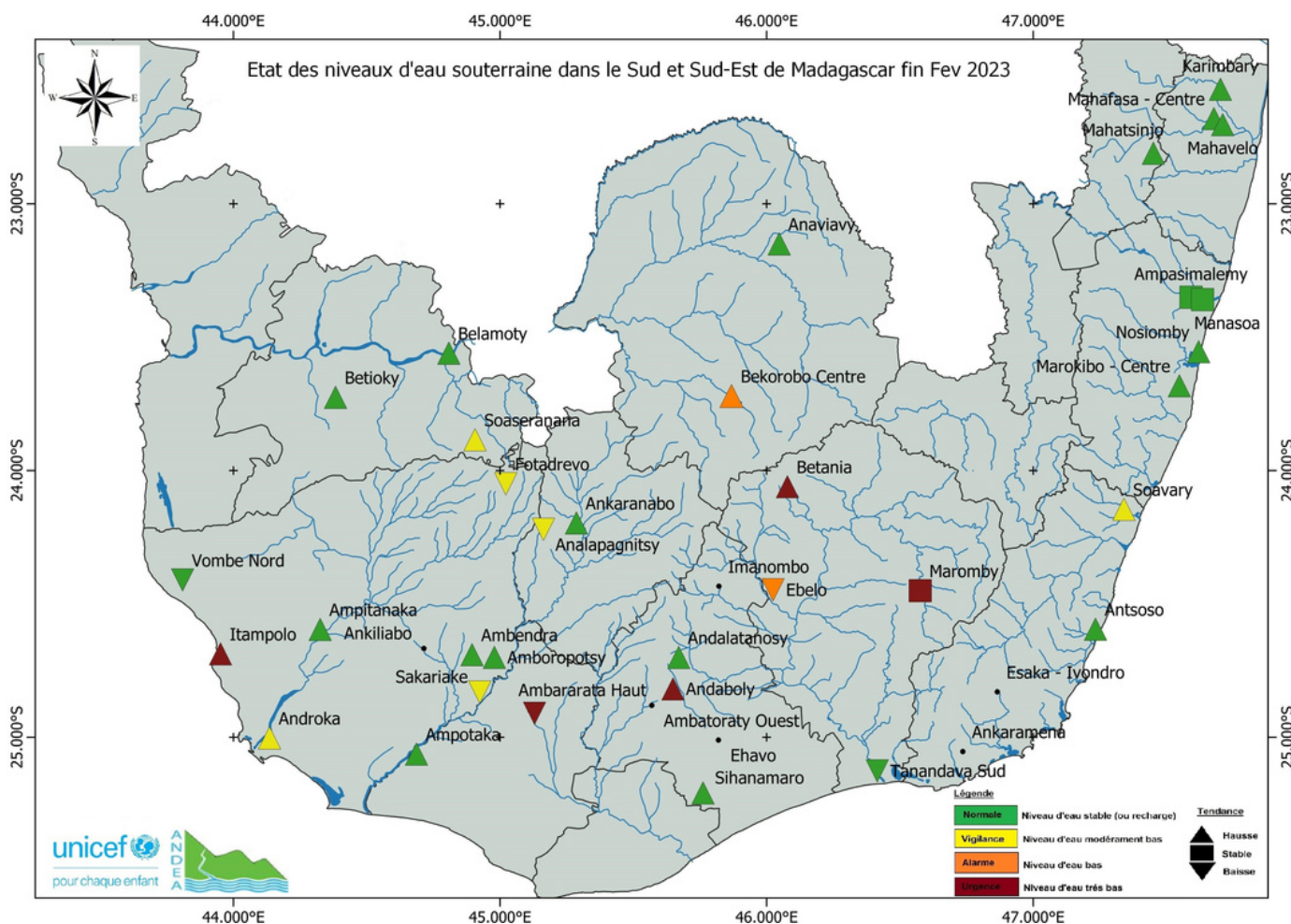
Fig. 2 Etat des niveaux d'eaux souterraines fin Fév 2023
