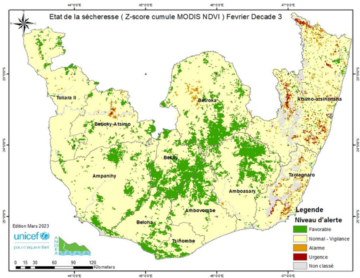
Fig. 1 : Etat de la sécheresse (anomalie zNDVIc) Fev Décade 3
